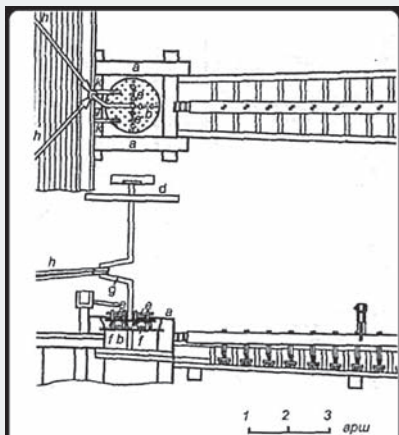
Рис. 27. Золотопромывальная машина Л. И. Брусницына
